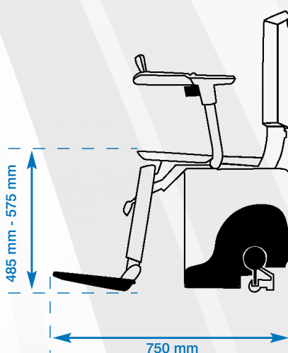
SEITENANSICHT – Aufgeklappt
