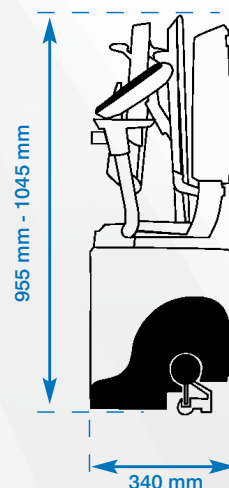
SEITENANSICHT – Zusammengeklappt
